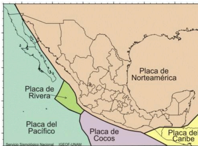
Figura 4. Placas tectónicas que interactúan en territorio mexicano
