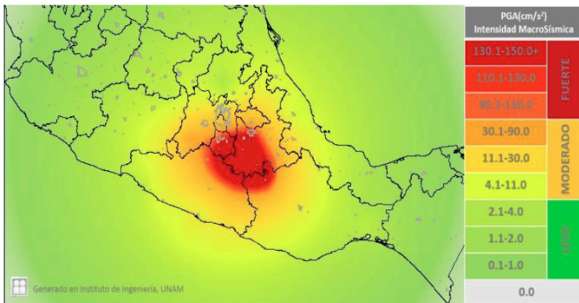
Figura 2. Mapa de intensidades del temblor del día 19 de septiembre de 2017.
