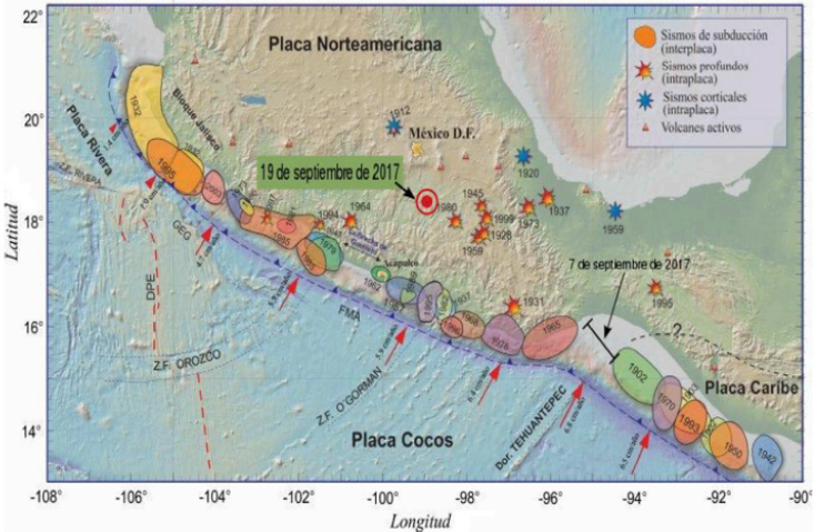
Figura 3. Áreas de ruptura de los sismos más importantes que han ocurrido en México. El epicentro del sismo del 19 de septiembre de 2017 se representa con un punto de color rojo.
